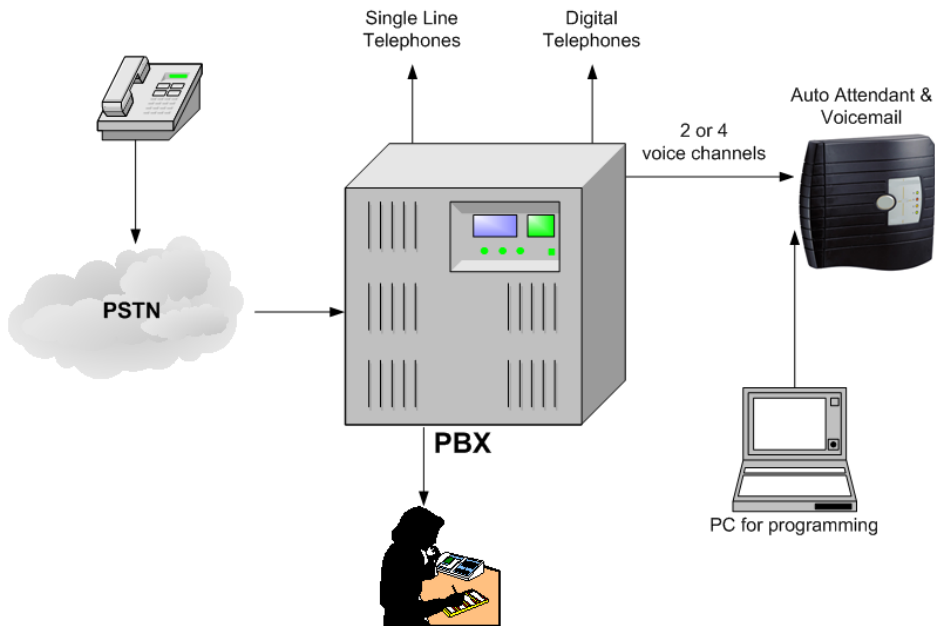
Рис. 2.5. Схема соединений Системы , УАТС и компьютера.
