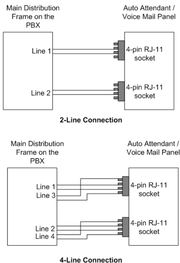
Рис. 2.4. Соединение Системы и УАТС.
