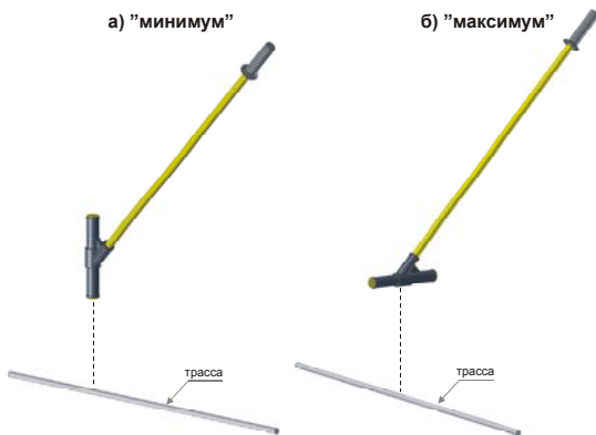
Рис 5. Положение антенны 45° над трассой при поиске по «минимуму»- а), и по «максимуму» - б).
