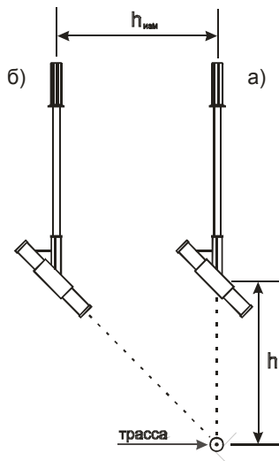
Рисунок 8. Определение глубины залегания трассы антенной 45°.
