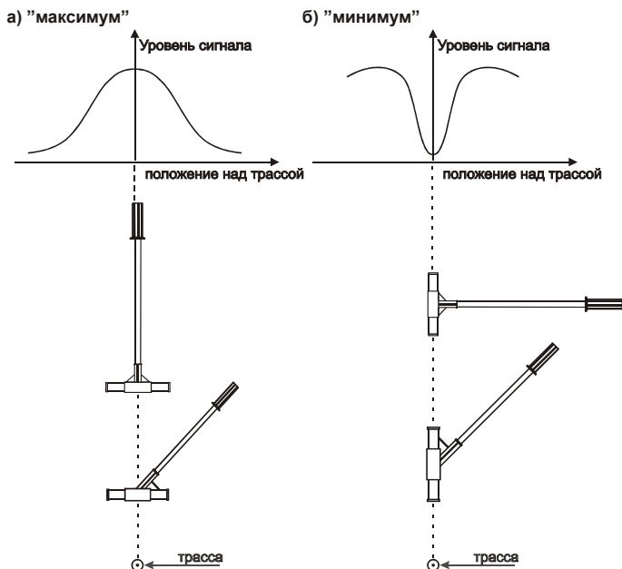
Рис. 6. Зависимость уровня сигнала от положения антенны над трассой и режима поиска.
