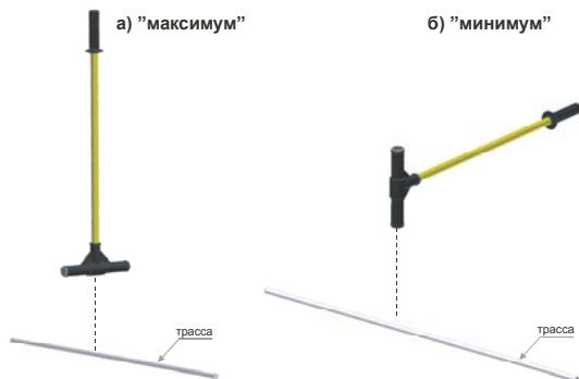
Рис 4. Положение антенны над трассой при поиске по «максимуму»- а), и по «минимуму» - б).
