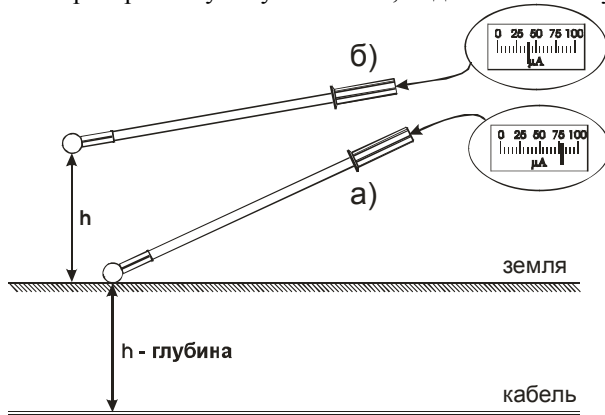
Рис. 7. Определение глубины трассы антенной 90^\circ .
